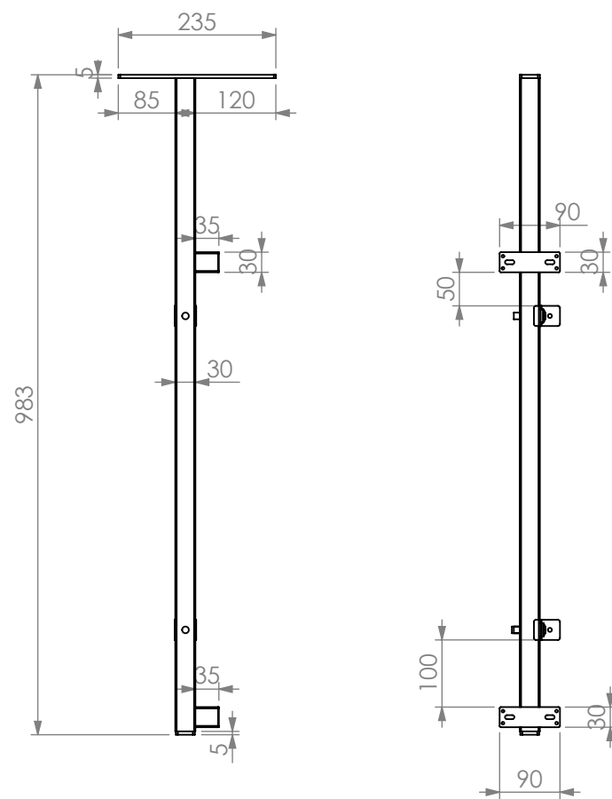
FRAME SCALE:1:12@A3
