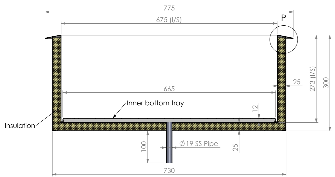
SECTION A-A
