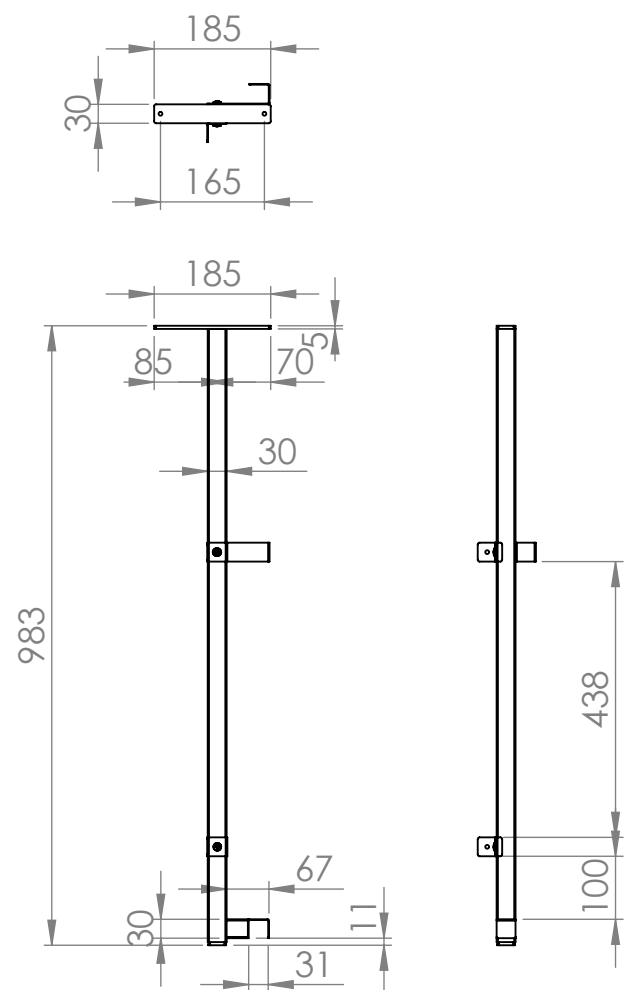
FRAME SCALE:1:12@A3
