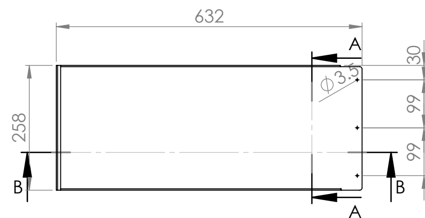
FRAME SCALE:1:12@A3
