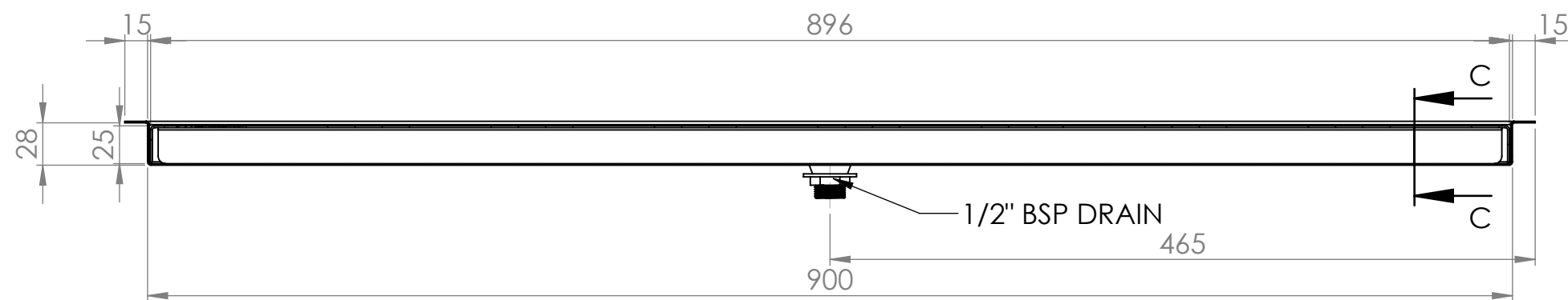
SECTION A-A
