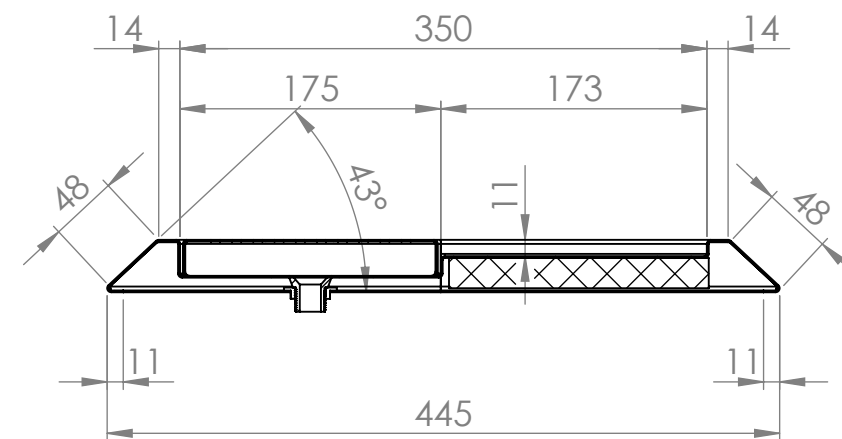
SECTION D-D
